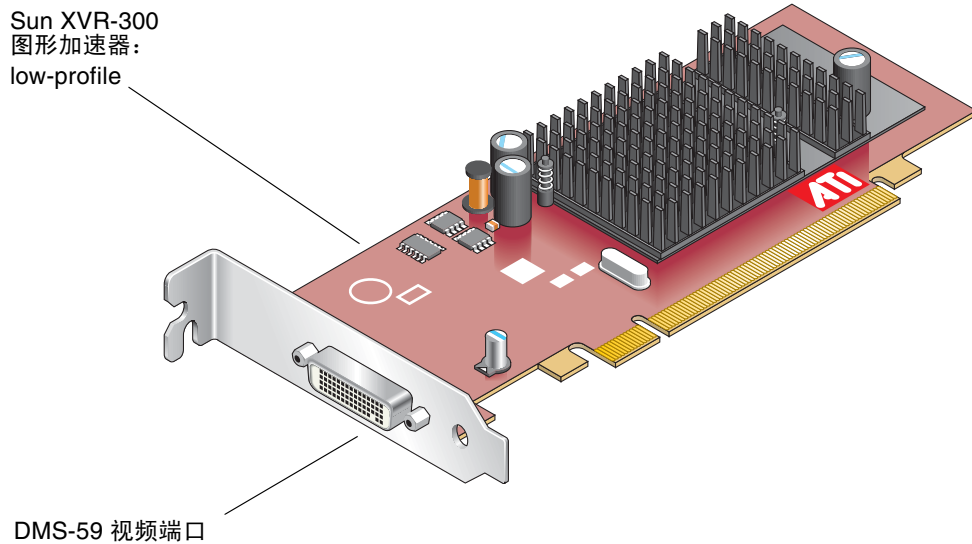
图 1-2 Low-Profile 型 Sun XVR-300 图形加速器
