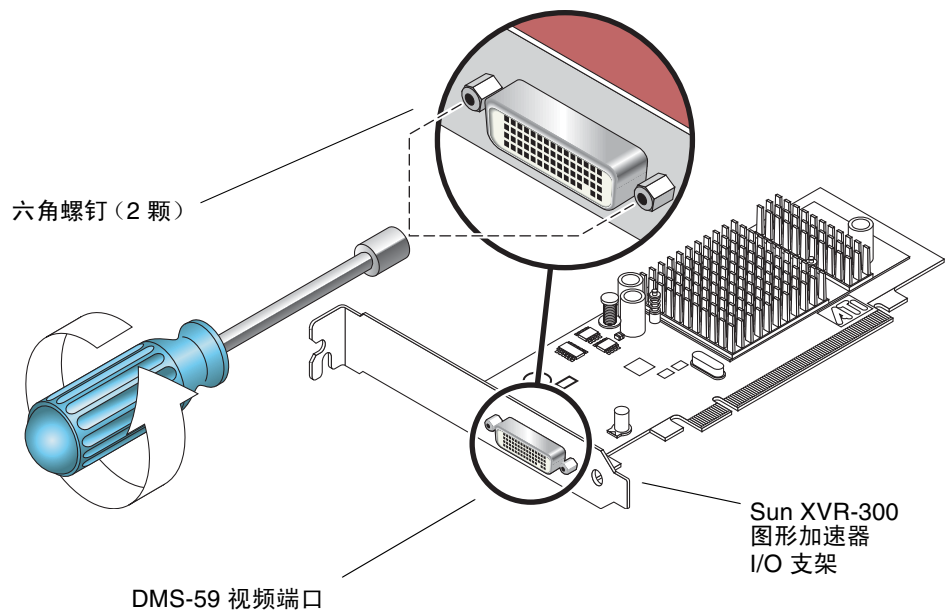
图 2-1 更换 I/O 支架
