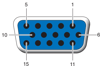
图 B-4 HD15 (VGA) 连接器
