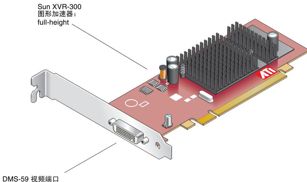
图 1-1 Full-Height 型 Sun XVR-300 图形加速器
