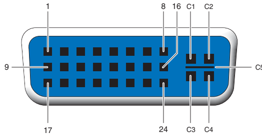
图 B-3 DMS-59 – 2xDVI-I 适配器分路器电缆 DVI 连接器
