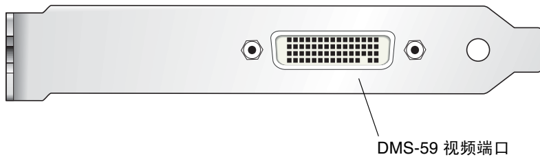
图 B-1 Sun XVR-300 图形加速器的 DMS-59 视频端口
