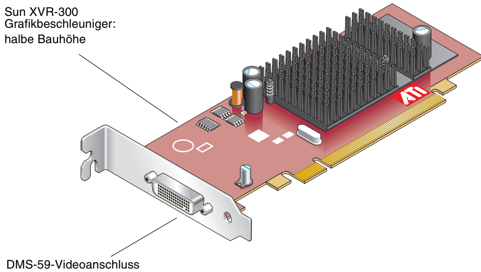
ABBILDUNG 1-2 Sun XVR-300-Grafikbeschleuniger, halbe Bauhöhe
