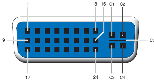
ABBILDUNG B-3 DMS-59 – 2xDVI-I Y-Kabeladapter DVI-Anschluss
