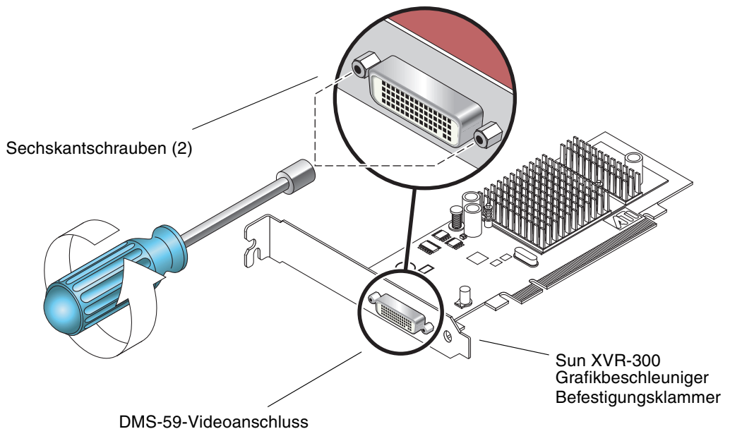
ABBILDUNG 2-1 Ersetzen der Befestigungsklammer
