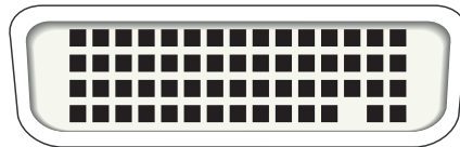
ABBILDUNG B-2 DMS-59-Anschluss
