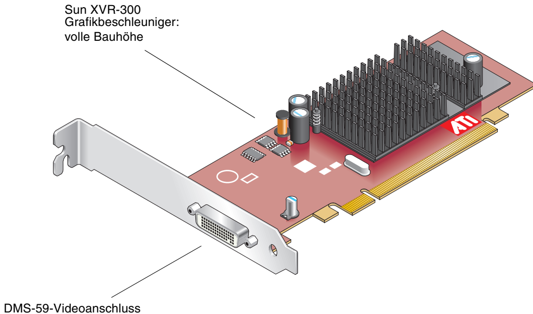
ABBILDUNG 1-1 Sun XVR-300-Grafikbeschleuniger, volle Bauhöhe
