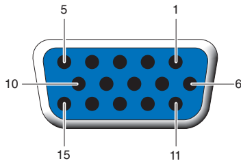
ABBILDUNG B-4 HD15 (VGA)-Anschluss
