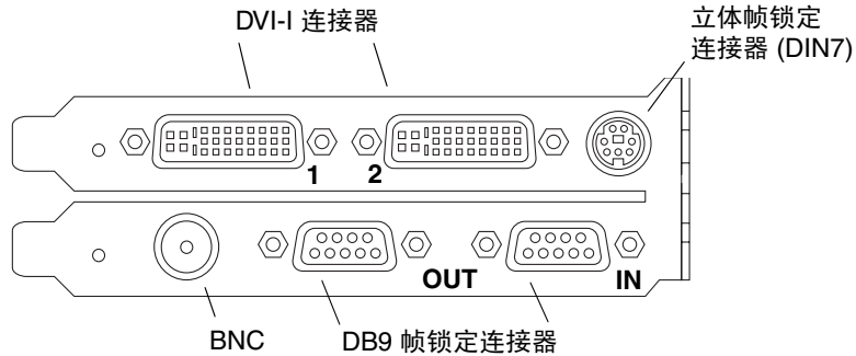
图 1-2 Sun XVR-1200 图形加速器后面板 I/O 端口
